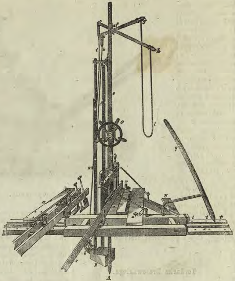
Fig. 5. Torfiarka Bróssowskiego.
